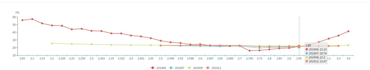
图 4 隐含波动率微笑
