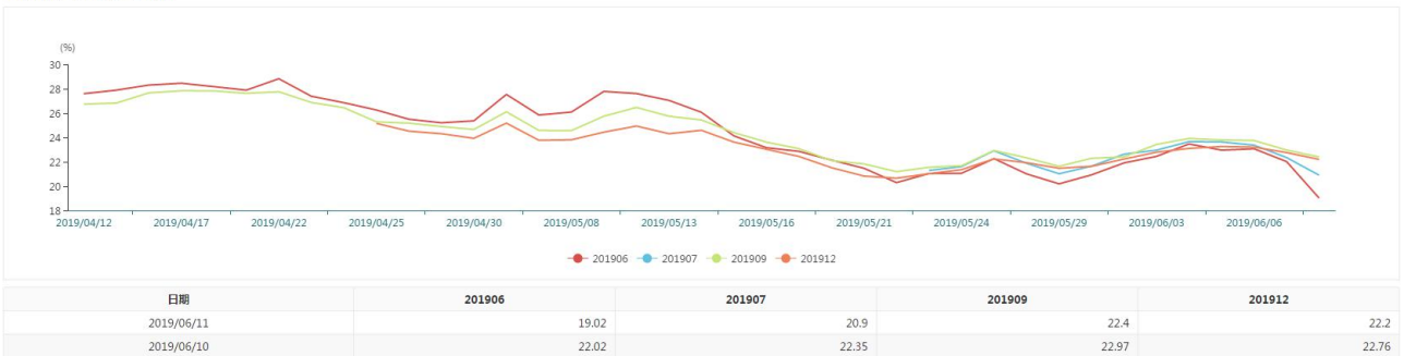
图 3 隐含波动率期限结构
