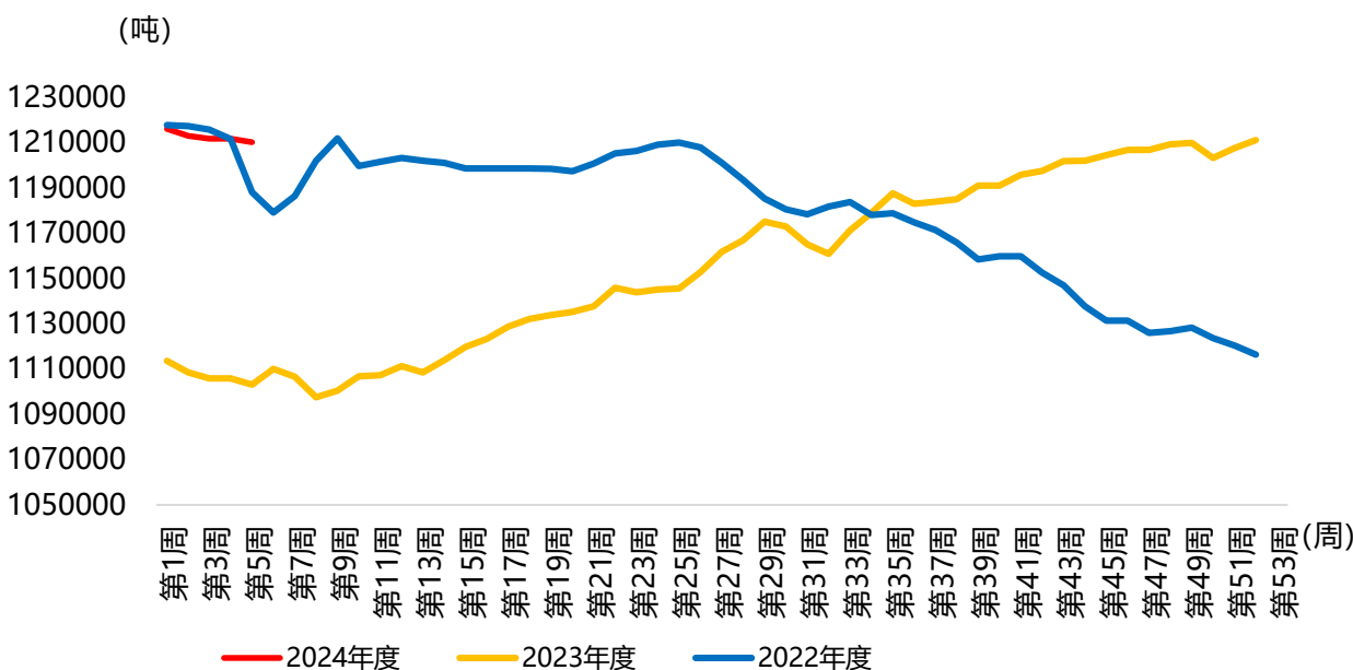
图 10 浮法玻璃周度产量
